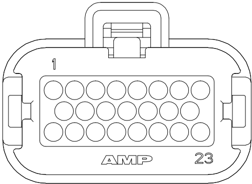
控制器接插件插线端子正视面
